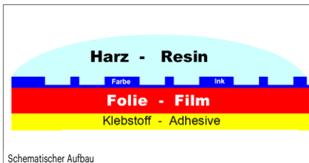
Schematischer Aufbau
